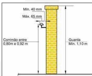
Dimensões de guardas e corrimãos
