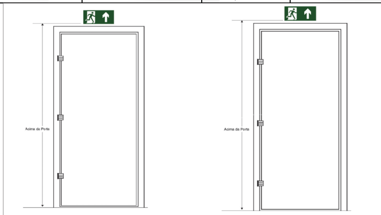
Figura C-5: Sinalização de portas com barras antipânico (modelos 1 e 2) da IT-20/2017
