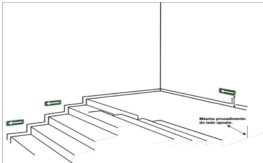
Figura C-8: Sinalização complementar da IT-20/2017. Exemplo de rodapé
