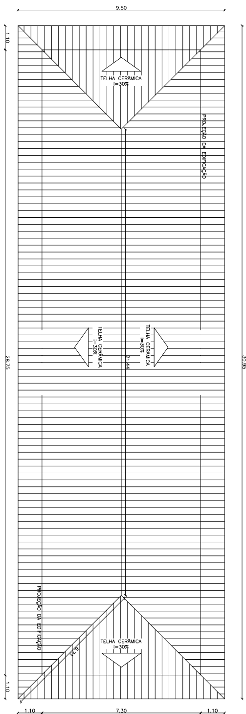
PLANTA DE COBERTURA - 1/100
