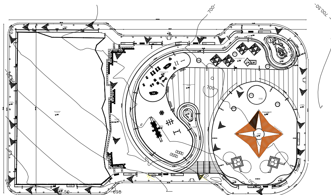
PLANTA DE DRENAGEM - ESCALA 1:150
