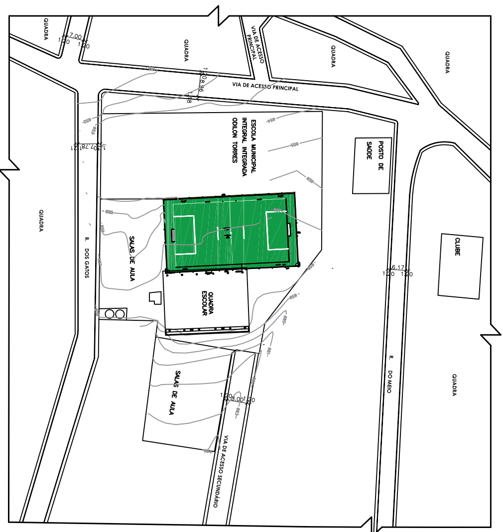
PLANTA DE SITUAÇÃO - ESCALA 1:1500
