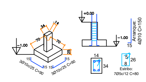
SAPATA QUADRADA P1 a P25 (TODOS)
