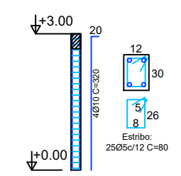
DETALHE PILAR (MORRE) P1 a P25 (TODOS)
