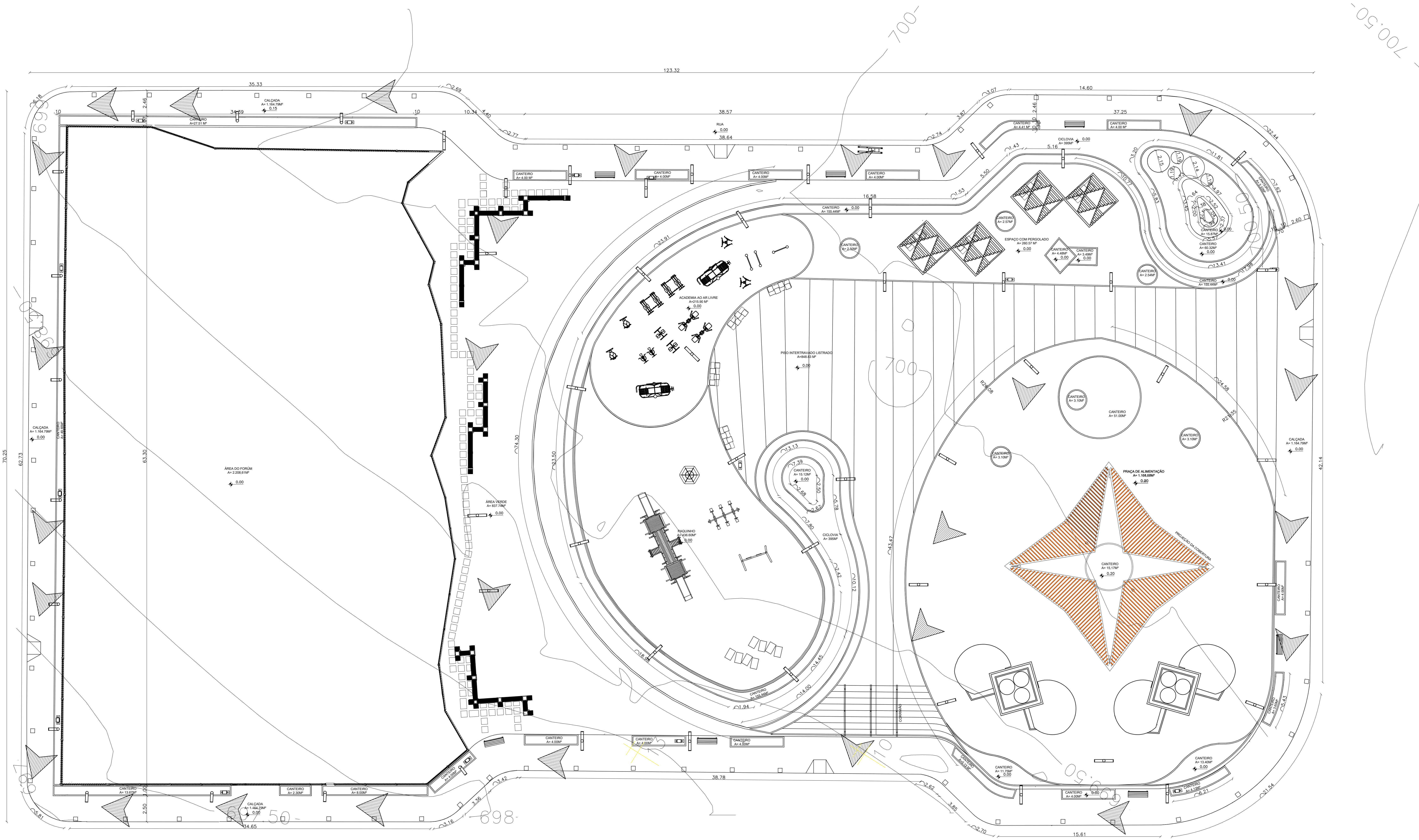
PLANTA DE DRENAGEM - ESCALA 1:150
