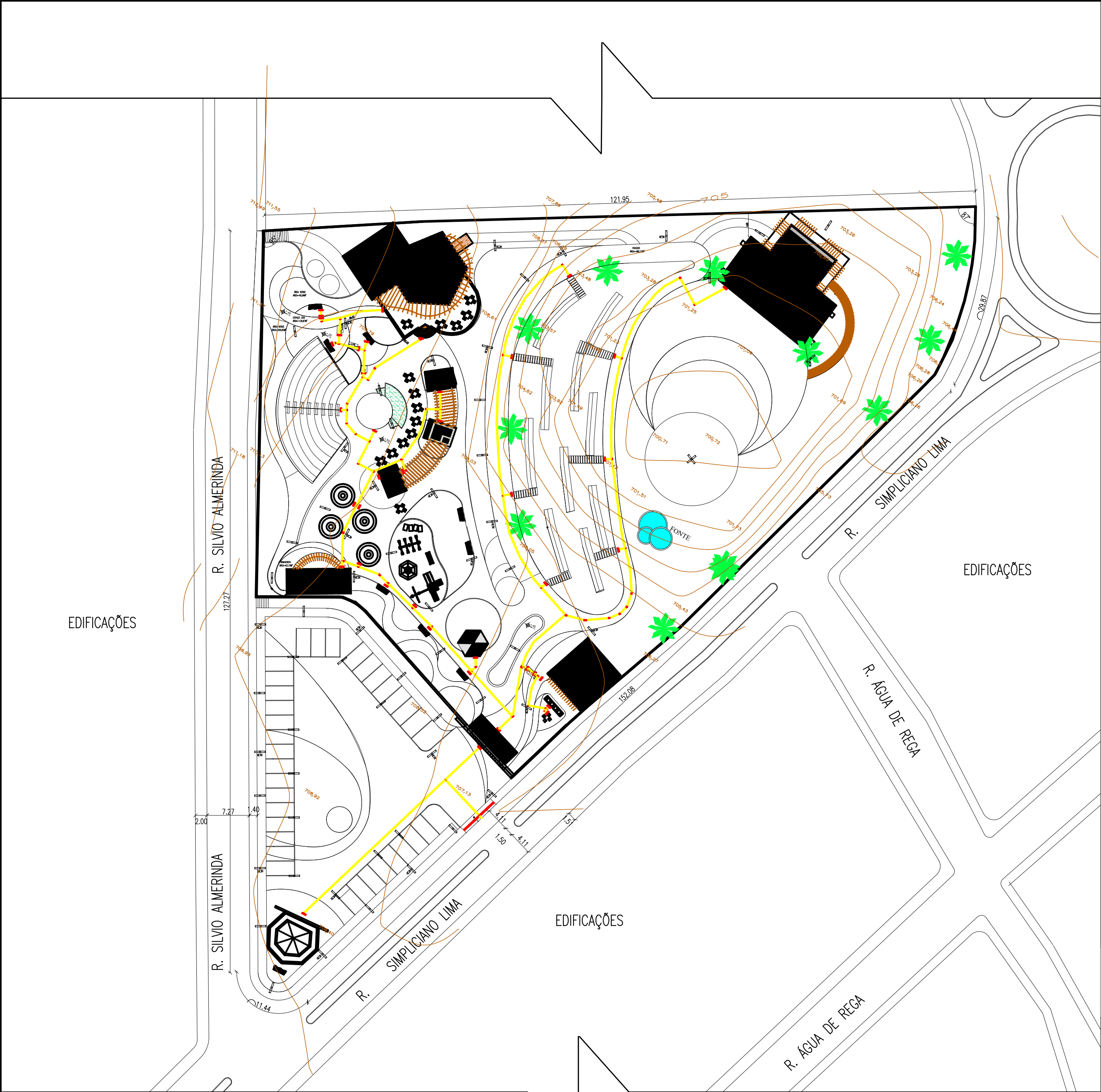
PLANTA DE IMPLANTAÇÃO – ESCALA 1:500
