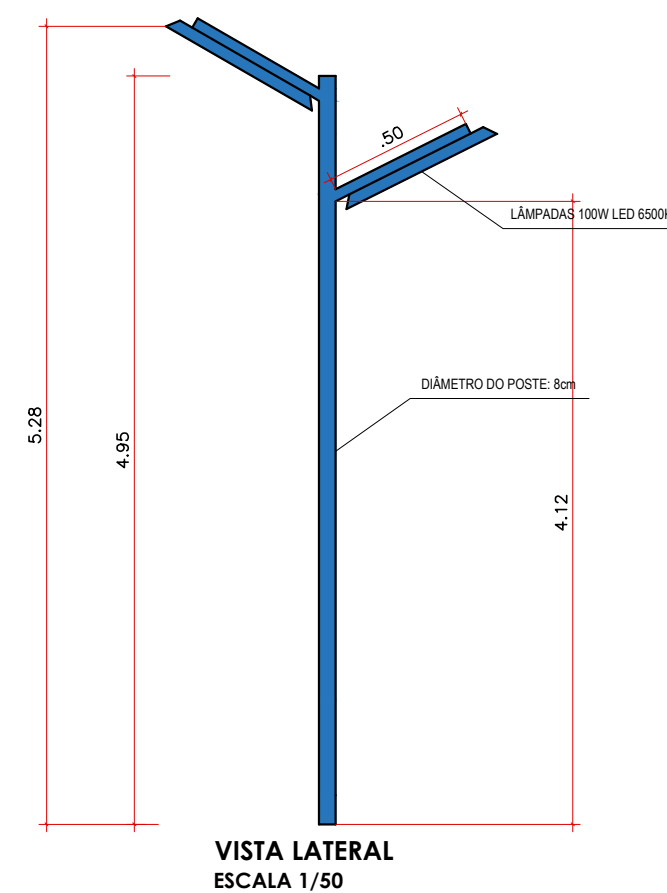
POSTE- ESCALA 1:50
