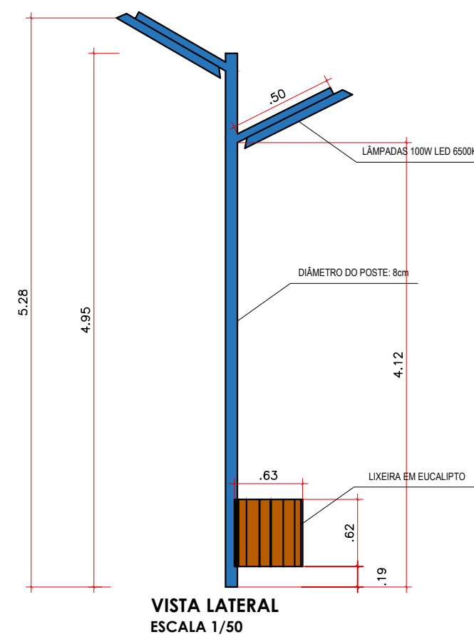
POSTE COM LIXEIRA - ESCALA 1:50
