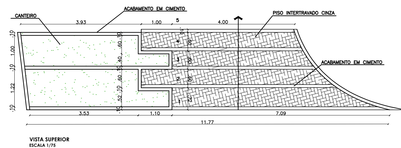
ESCADA COM CANTEIRO- ESCALA 1:75
