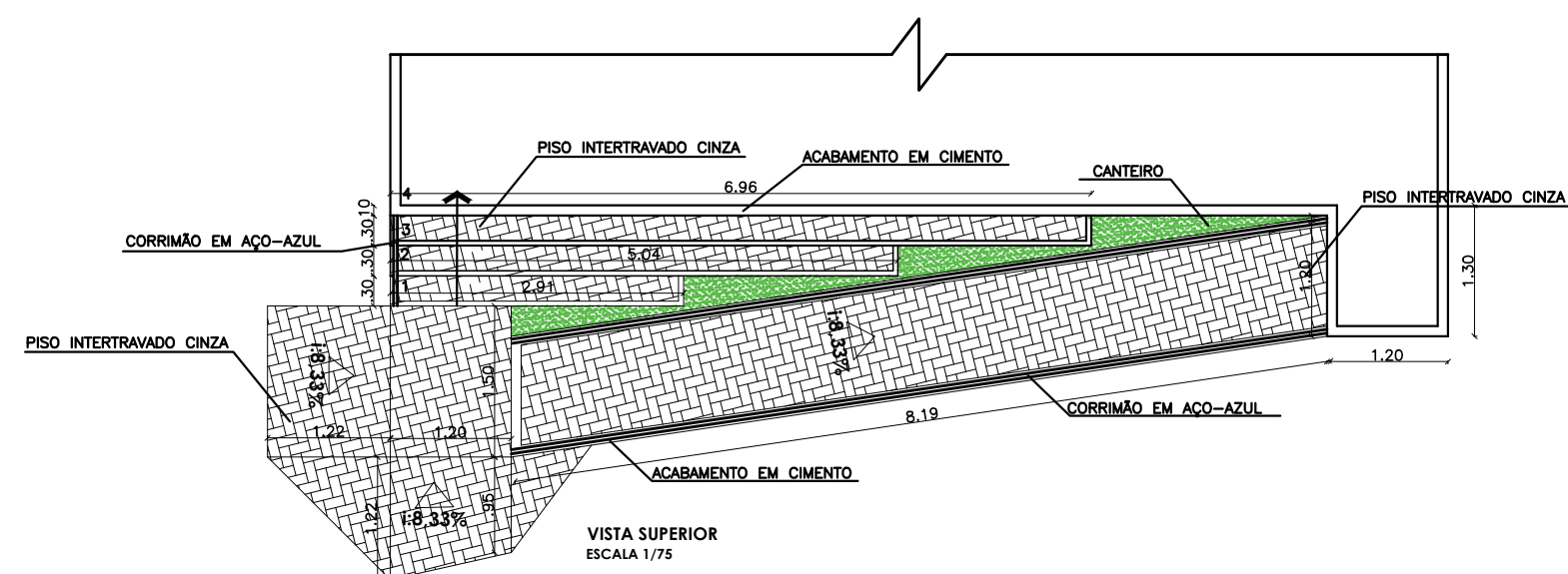
ESCADA COM RAMPA - ESCALA 1:75
