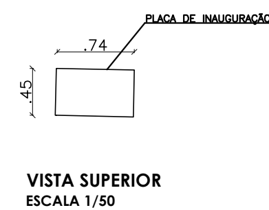
SUPORE PARA PLACA - ESCALA 1:50
