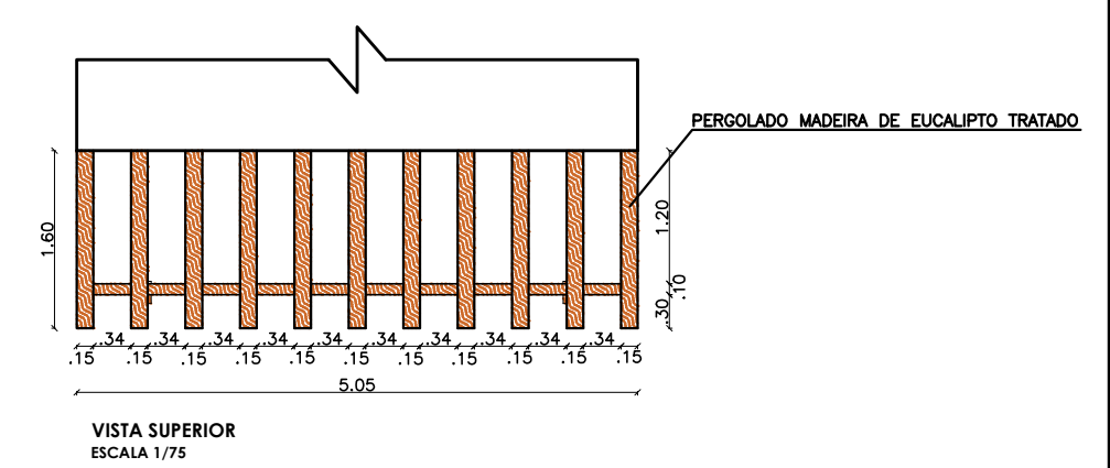
PERGOLADO EM MADEIRA 01 - ESCALA 1:75
