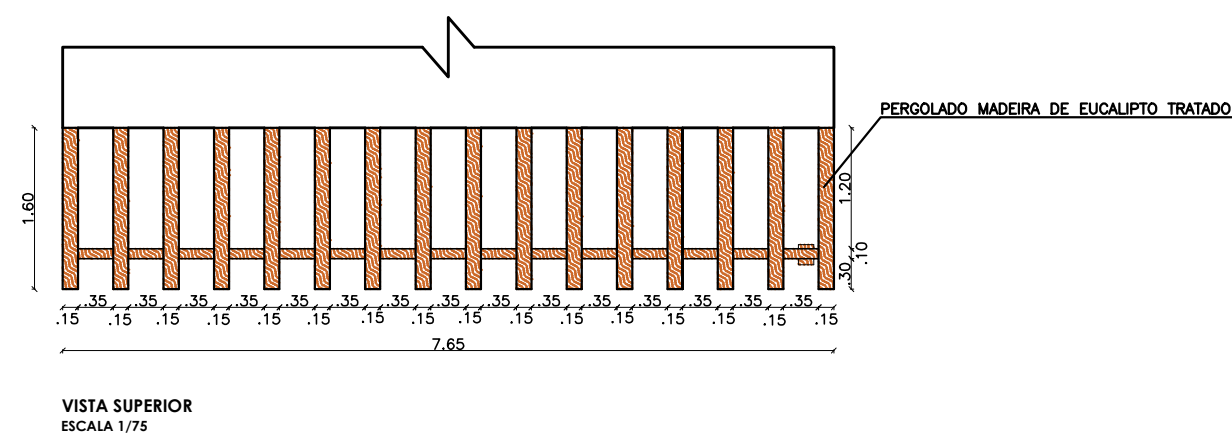
PERGOLADO EM MADEIRA 02 - ESCALA 1:75
