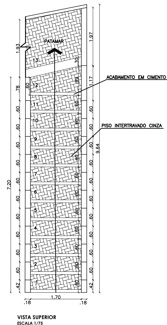
ESCADA - ESCALA 1:75
