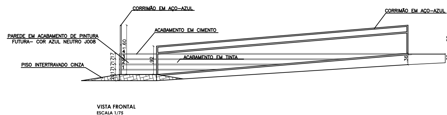
ESCADA COM RAMPA - ESCALA 1:75
