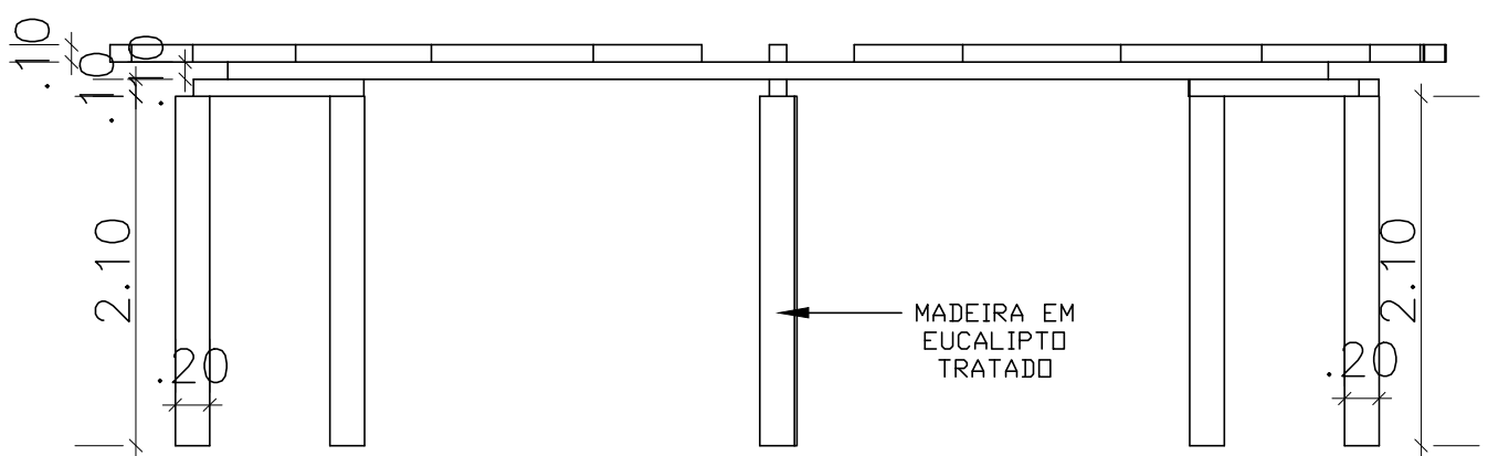
VISTA LATERAL PERGOLADO CIRCULAR ESCALA 1:50
