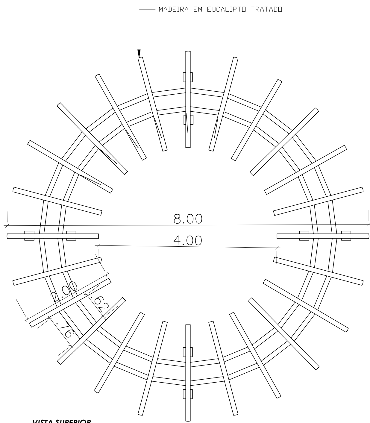
VISTA SUPERIOR PERGOLADO CIRCULAR ESCALA 1:50
