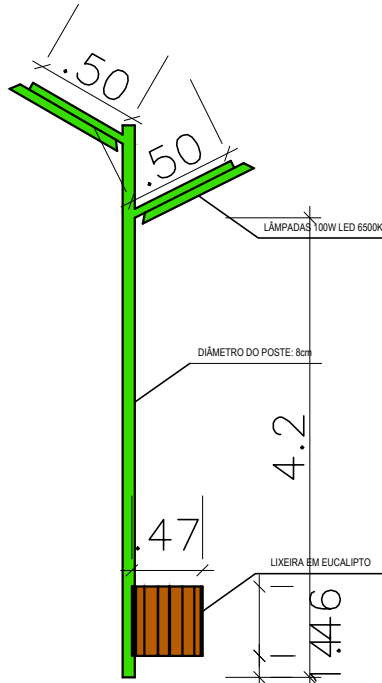
VISTA LATERAL POSTE DE ILUMINAÇÃO ESCALA 1:50
