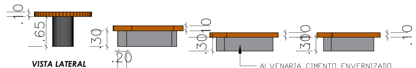
VISTA LATERAL MODELOS DE MESA E BANCOS ESCALA 1:50
