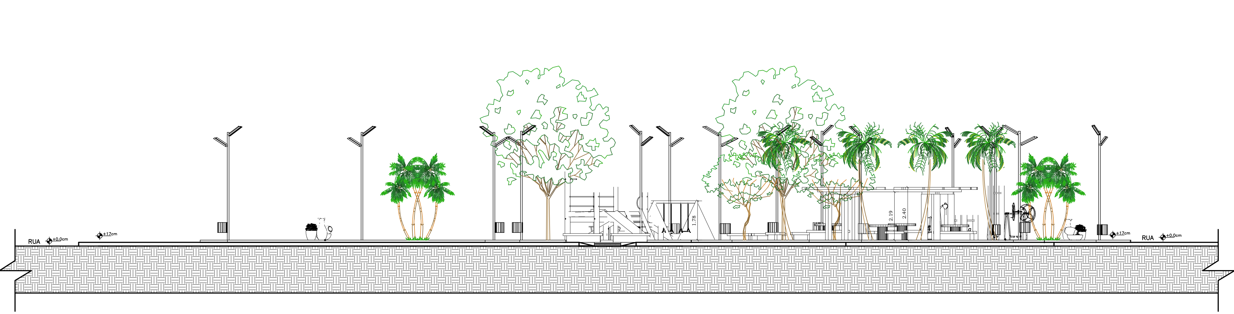
PERFIL C - ESCALA 1:100
