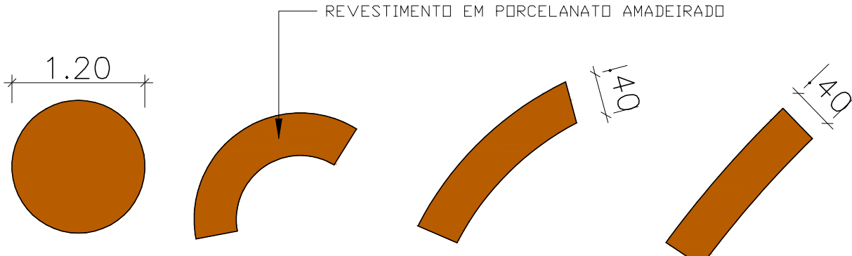
VISTA SUPERIOR MODELOS DE MESA E BANCO ESCALA 1:50
