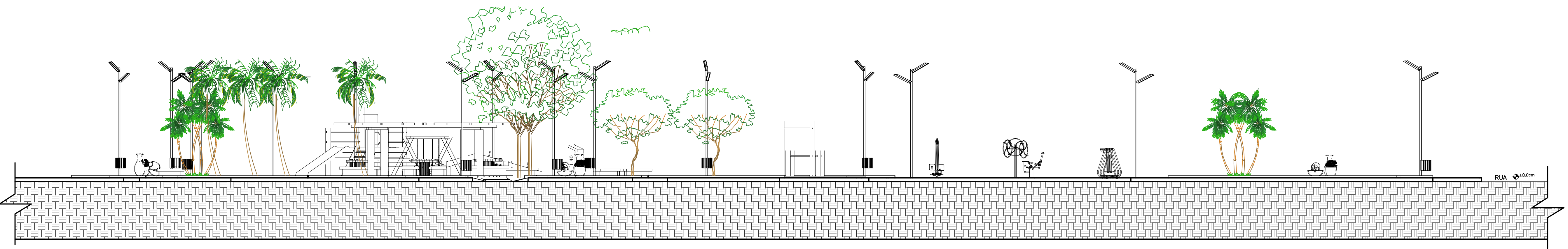
PERFIL B - ESCALA 1:100
