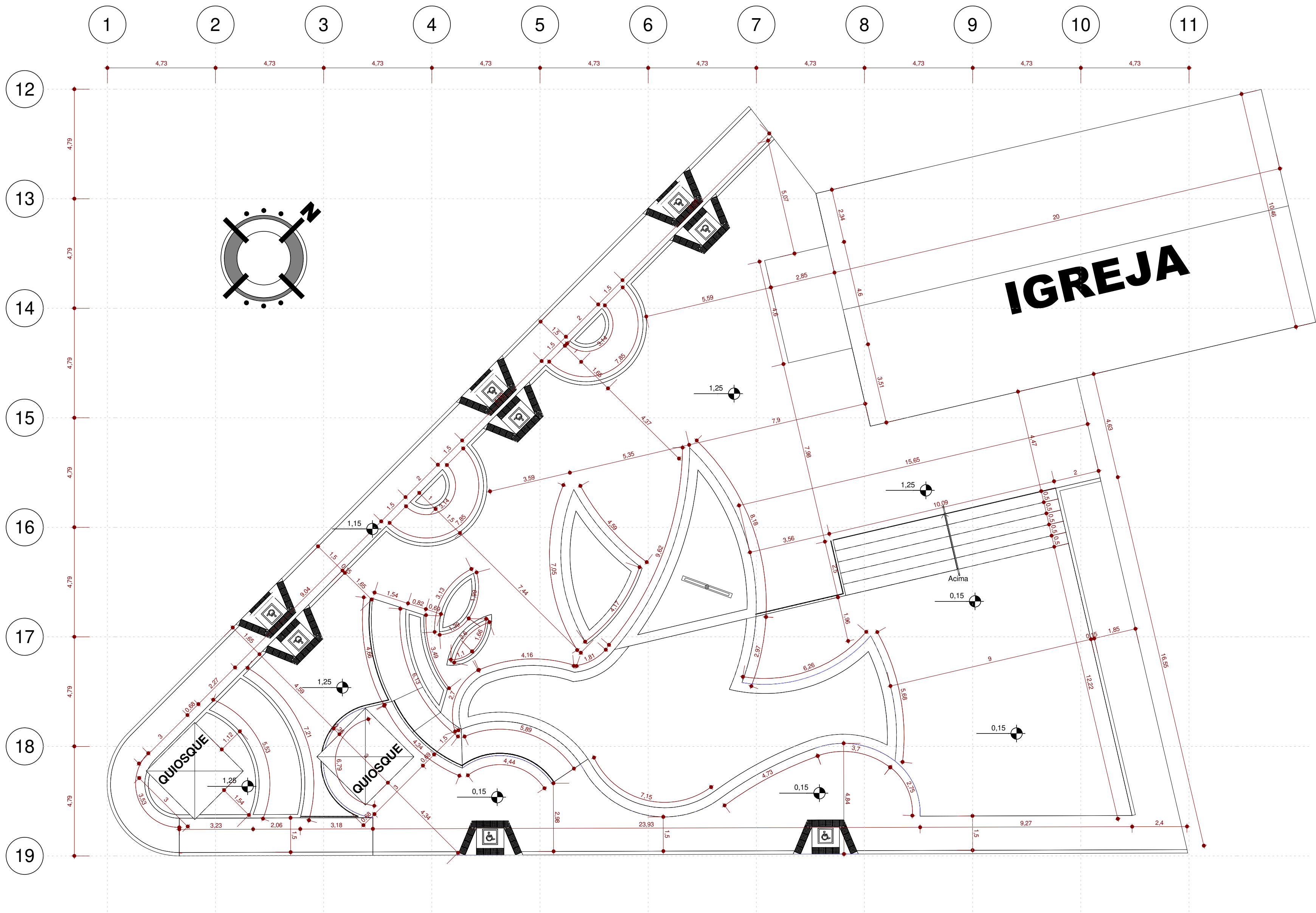
1 PLANTA DE COTAS ESCALA - 1 : 125
